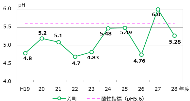
■ 降雪中の pH 値の推移
