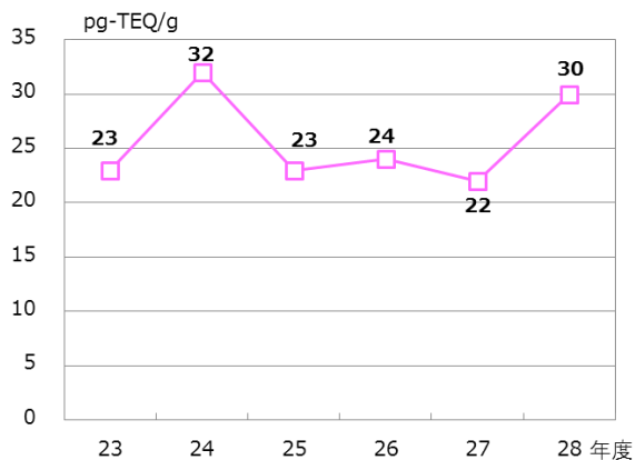
■ 清掃事業所周辺土壌のダイオキシン類濃度
