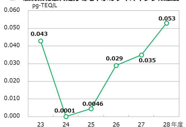
■ 一般廃棄物最終処分場地下水のダイオキシン類濃度
