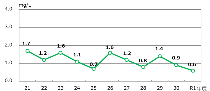
■ 広瀬川のBOD値（平均値）の経年変化
