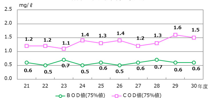
■ 入畑ダムの水質経年変化
