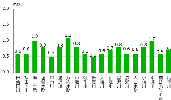
■ 令和元年度中小河川のBOD値（平均値）
