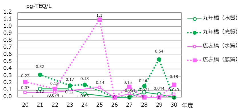
■ ダイオキシン類濃度調査結果（岩手県）
