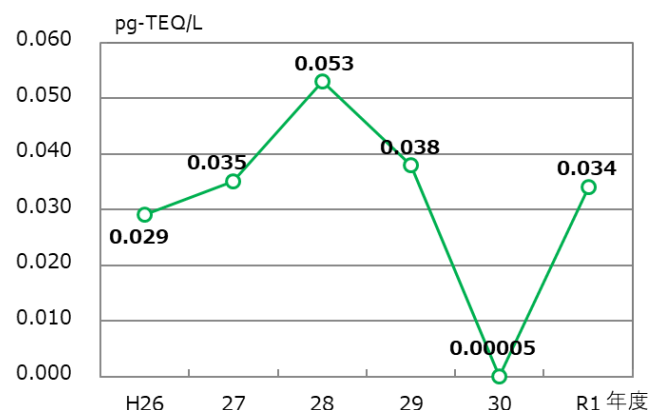
■ 一般廃棄物最終処分場地下水のダイオキシン類濃度
