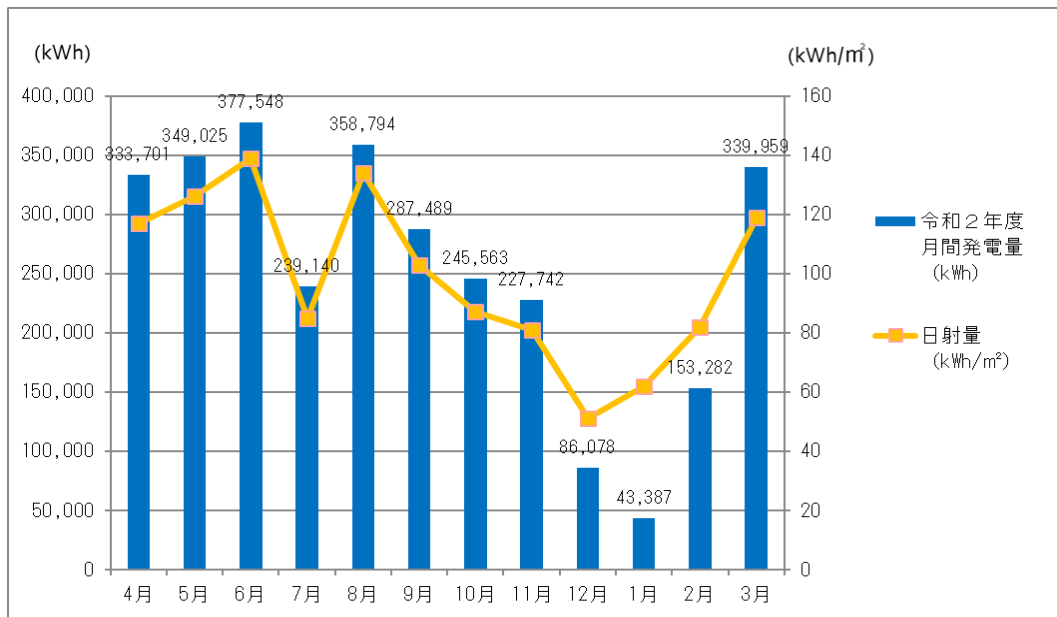
■ 令和2年度（かむいソーラー発電所）月別発電量（kWh）
