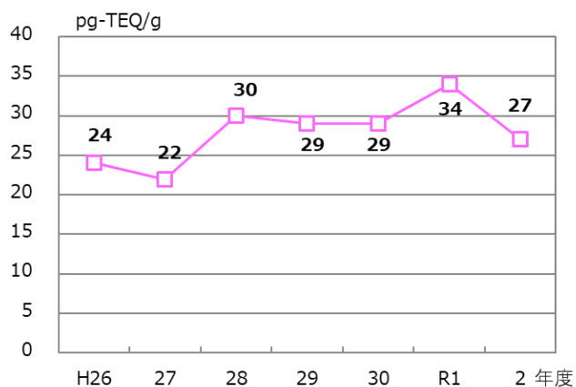
■ 清掃事業所周辺土壌のダイオキシン類濃度
