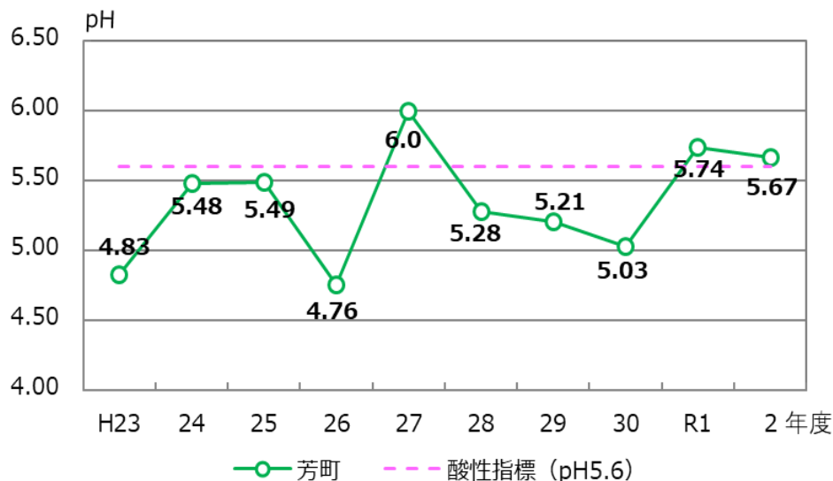
■ 降雪中の pH 値の推移
