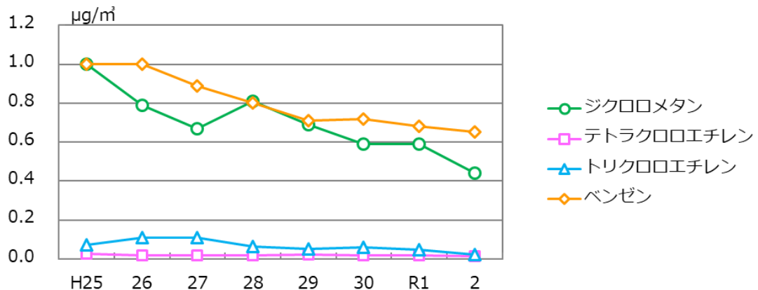
■ 環境基準設定項目の経年変化（芳町）
