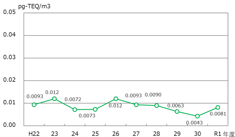
■ 一般環境地域のダイオキシン類毒性等量濃度経年変化
