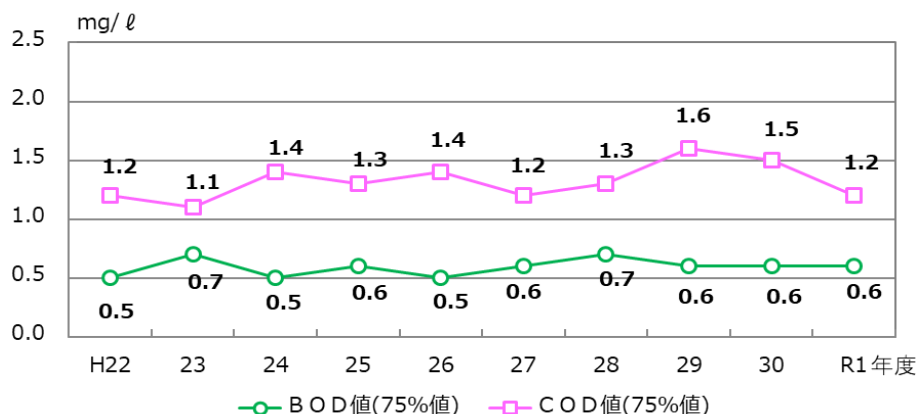
■ 入畑ダムの水質経年変化
