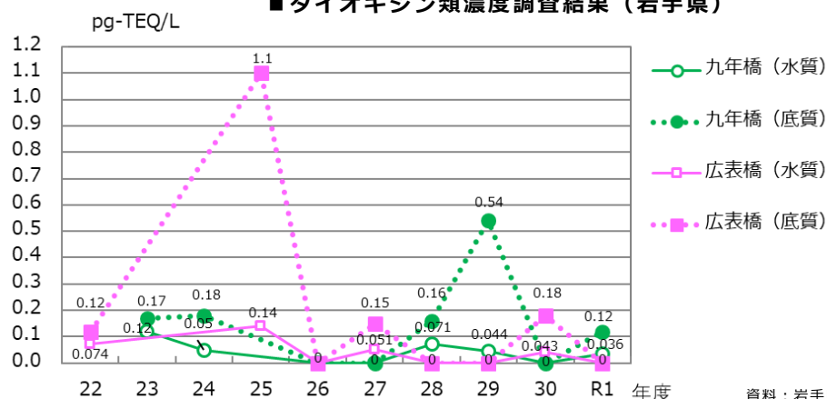
■ ダイオキシン類濃度調査結果（岩手県）
