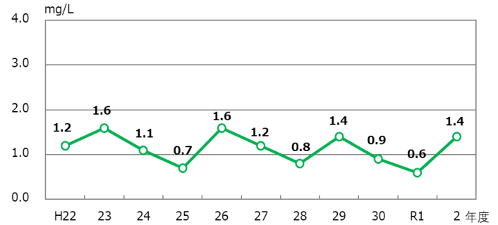
■ 広瀬川のBOD値（平均値）の経年変化
