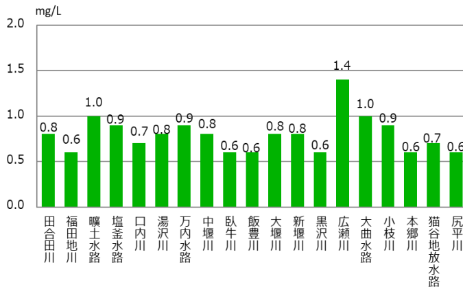
■ 令和2年度中小河川のBOD値（平均値）
