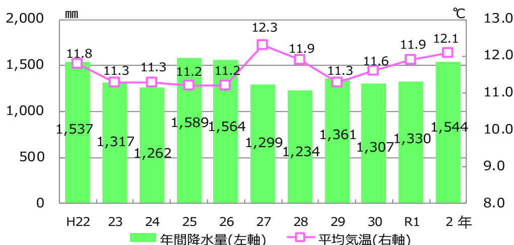
■ 年度別降水量と平均気温
