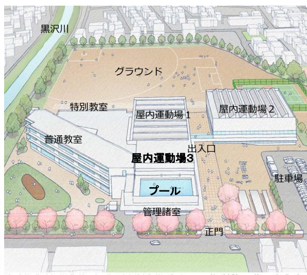
基本計画の配置(案)
